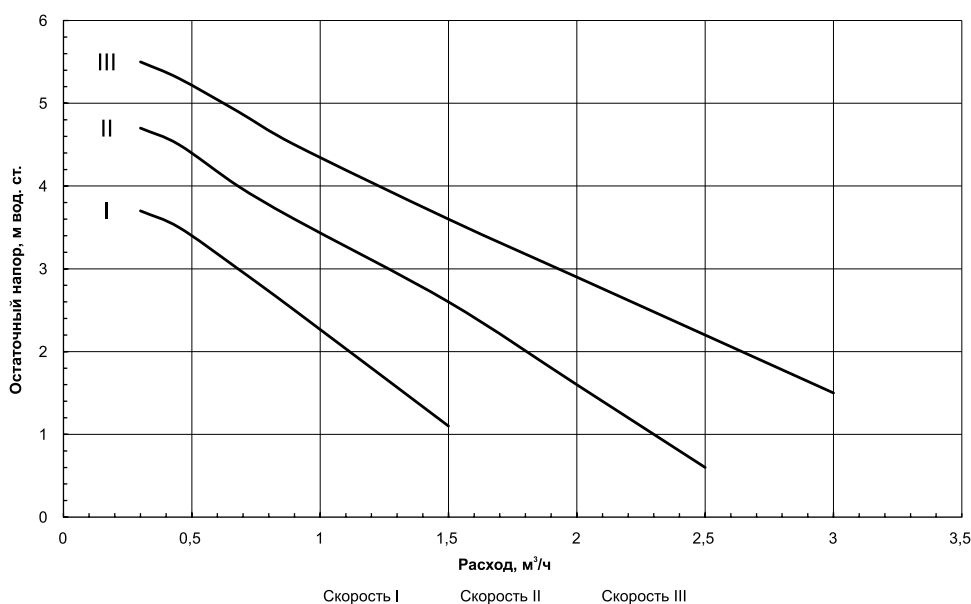
Рис.1.1 Остаточный напор для циркуляционного насоса ZOTA Ring 25/70 (Для котлов MK-S Plus 24-36)
